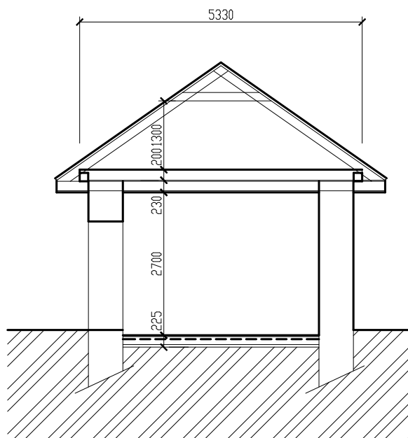
REZ A-A
