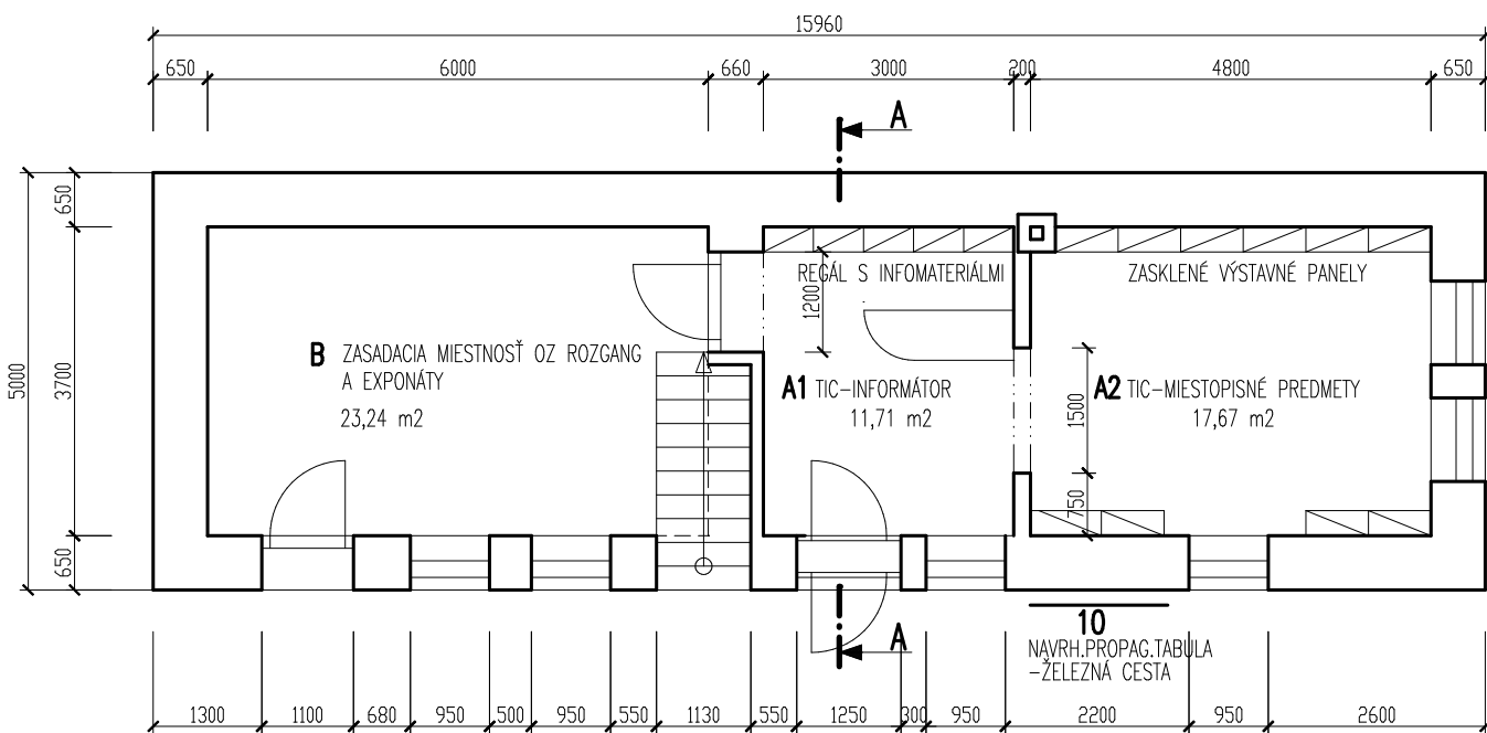
Pôdorys
